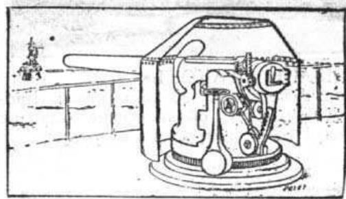
Скорострѣльная морская пушка Армстронга
