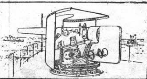
Скорострѣльная морская пушка Круппа на скользящемъ лафетѣ.
