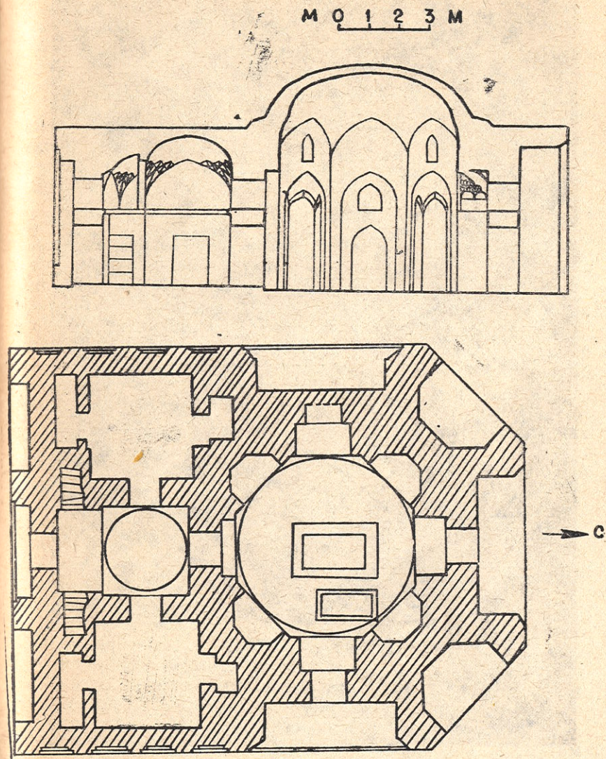
Рис. 22. План и разрез мазара Мири Рузадор (снят Г. А. Пугаченковой).
