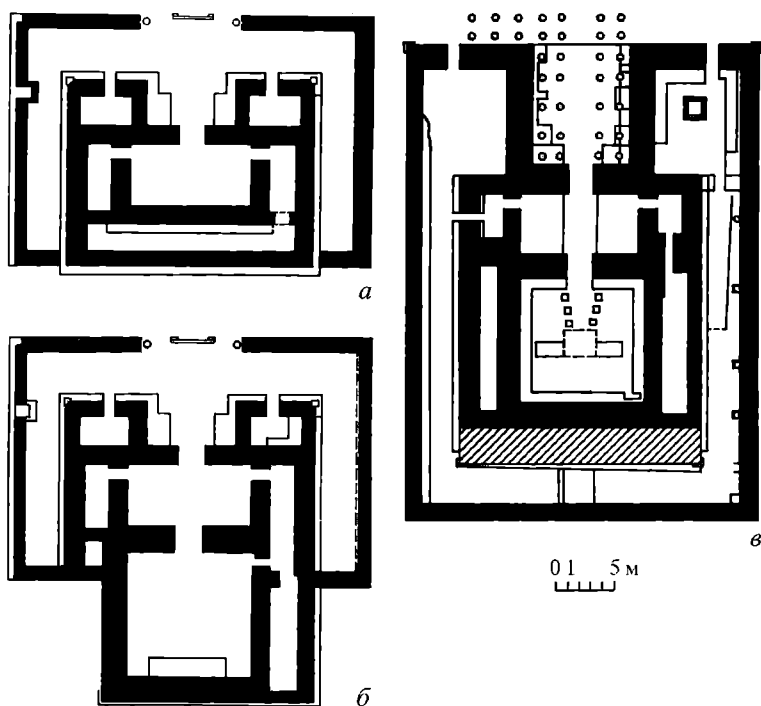
Рис. 9. Дильберджин. Храм Диоскуров. а – первый строительный период; б – второй строительный период; в – третий строительный период (по: Кругликова 1986)
