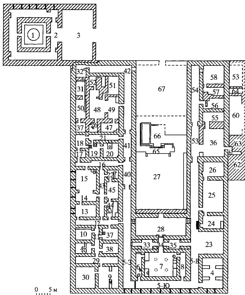
Рис. 13. Дильберджин. «Большой дом» и сардоба. План (по: Кругликова, Пугаченкова 1977)
