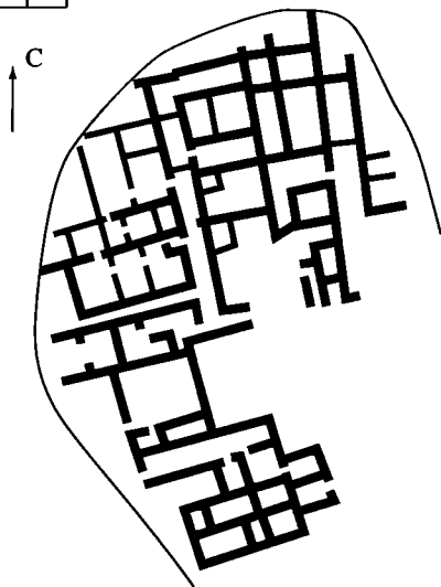
Рис. 5. Джагат-тепе. Западный блок жилых построек на поселении (по: Пугаченкова 1979)
