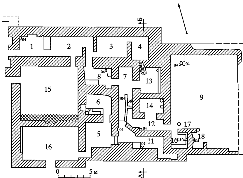
Рис. 14. Дильберджин. «Дом ремесленника». План (по: Крутликowa, Пугаченкова 1977)
