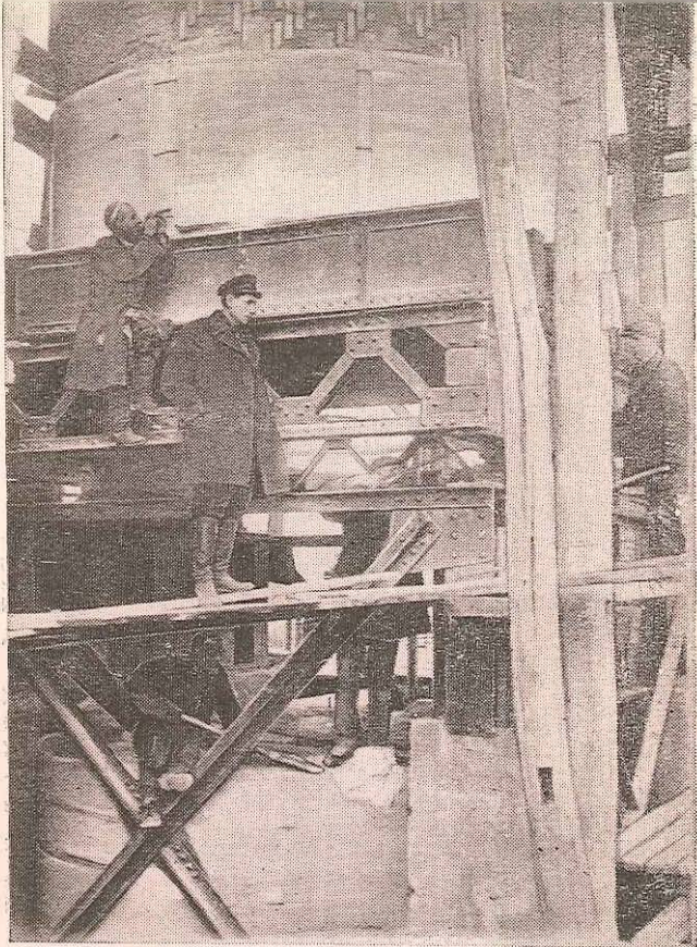
Металлическая конструкция в основании северо-восточного минарета медресе Улугбека (1932 г.). На переднем плane техник Г. И. Соловьев.
