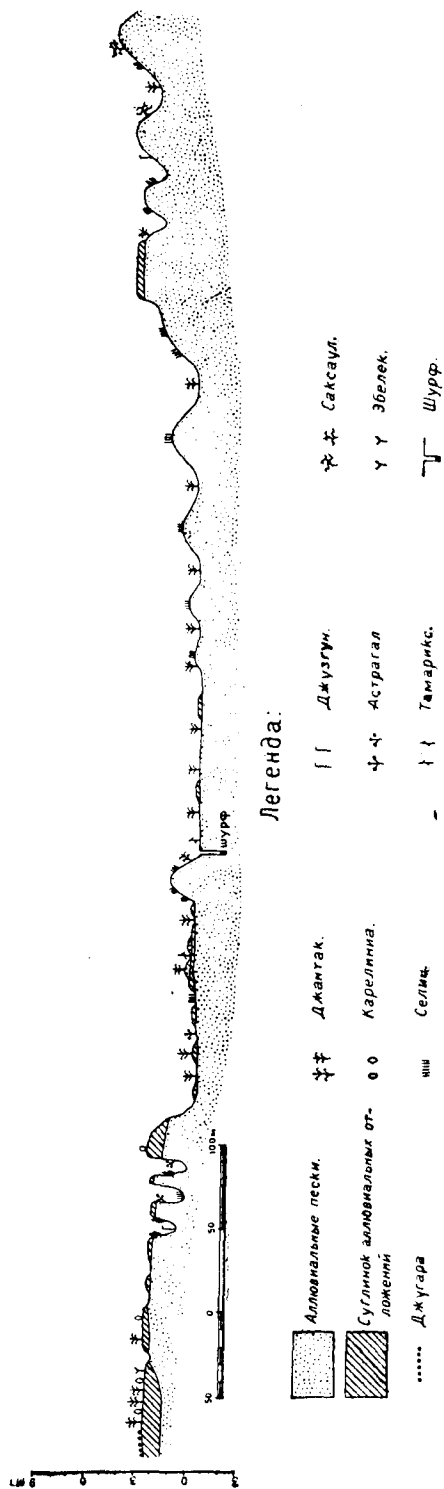
Схематический профиль полосы дефляции уроч. Гульдурсен.
