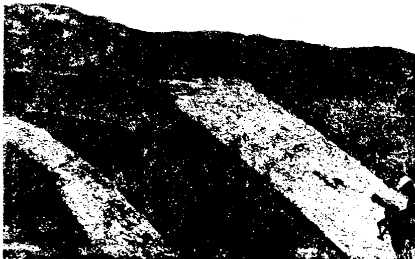
Кзыл-кумы. Пегматитовые жилы в граните Алтын-тау.
