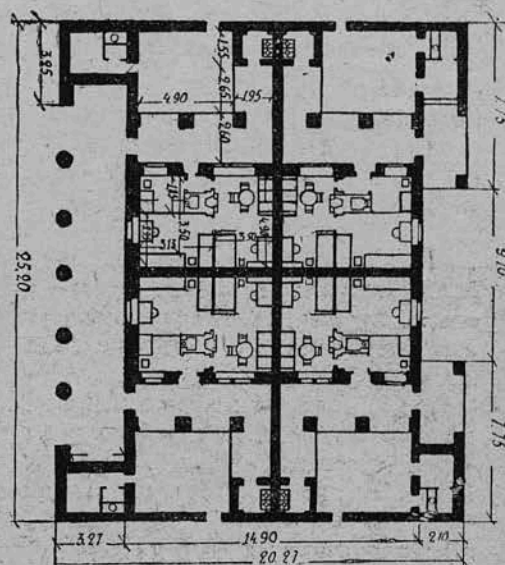
7. План четырехквартирного жилого дома
