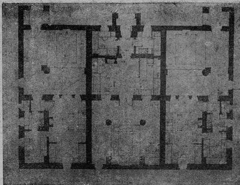
19. План трехквартирного дома
