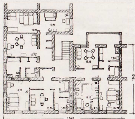
Угловая секция 3-2-3 Жилая площадь 132,94 м 2 Полезная площадь 200,98 м 2 Строительный объем 1021,8 м 3
