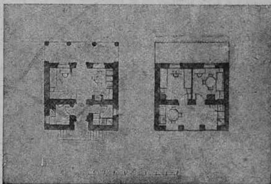
24. План двухэтажного одноквартирного дома
