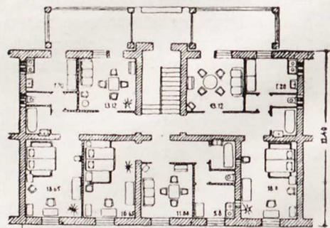
Рядовая секция 2-2-2 Жилая площадь 91,42 м 2 Полезная площадь 150,16 м 2 Строительный объем 748,5 м 3
