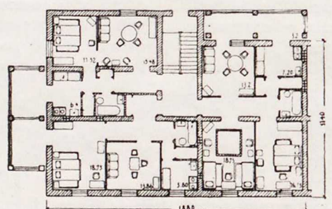
Торцовая секция 2-2-3 Жилая площадь 108,23 м 2 Полезная площадь 168,99 м 2 Строительный объем 862,56 м 3
