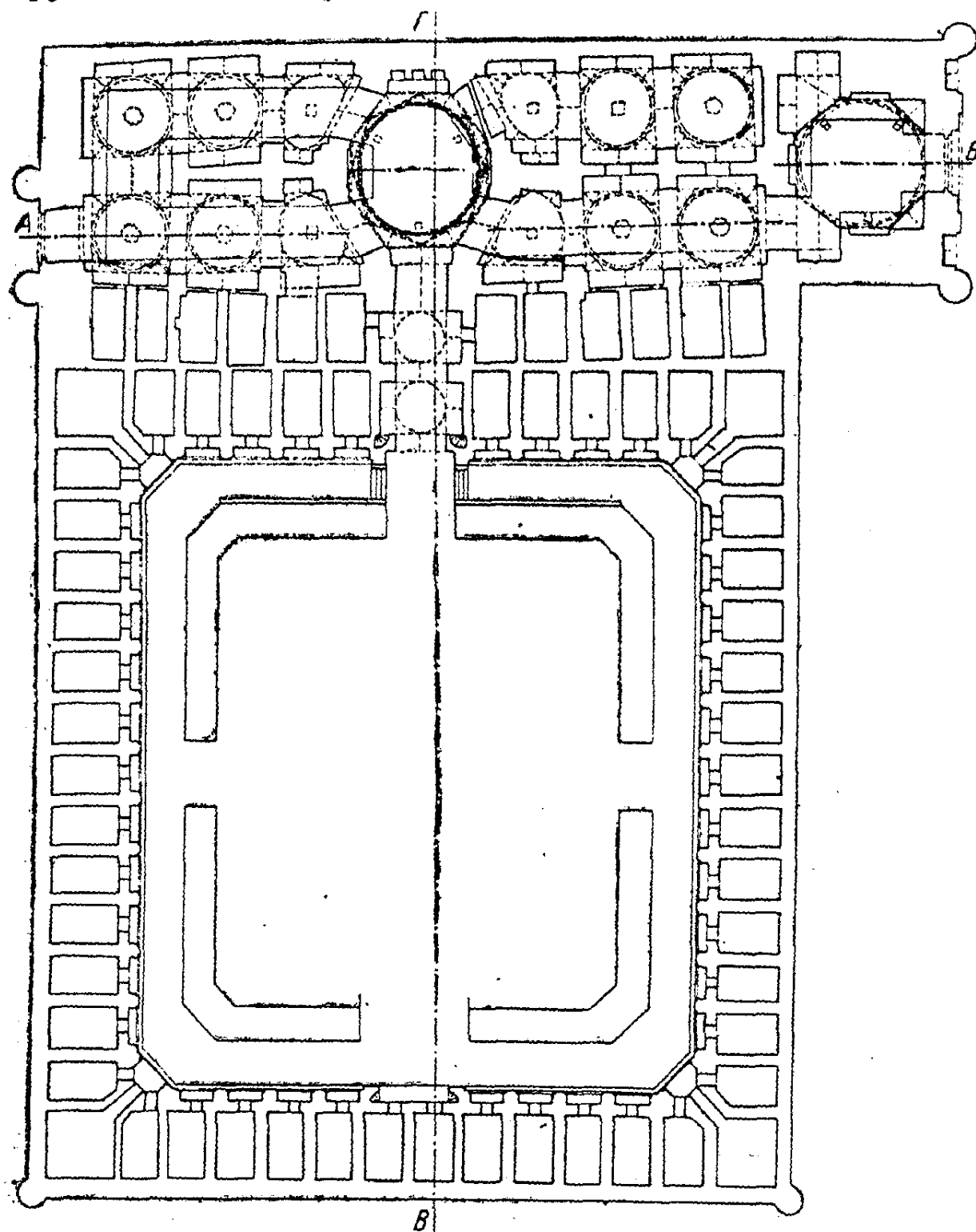
Рис. 18. План медресе Алла-Кули-хана
