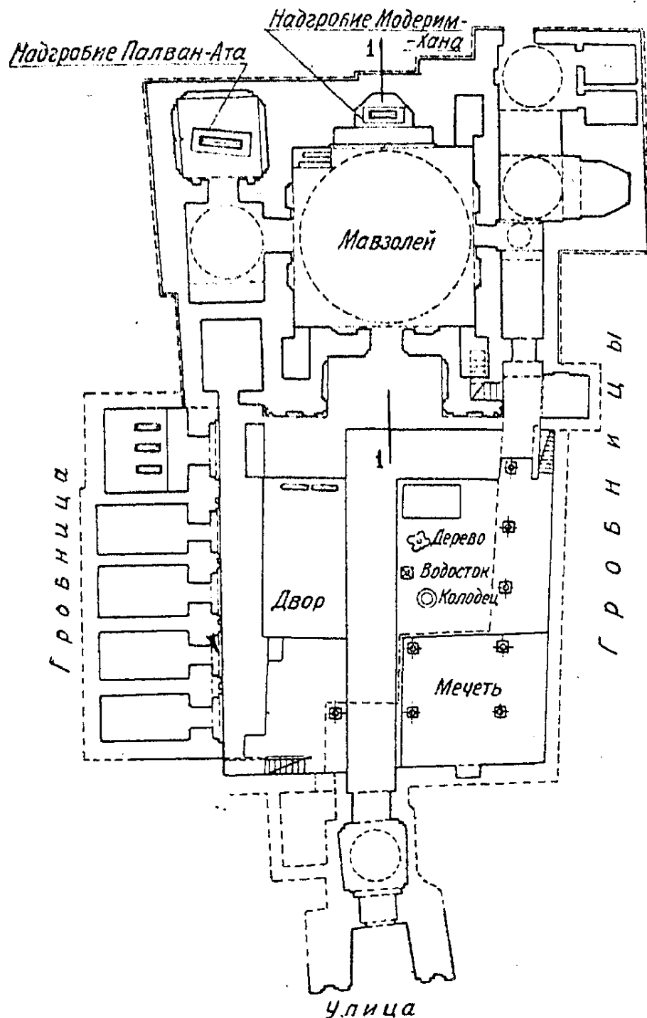
Рис. 15. План гумбе́за Пахлаван-Махмуда.
