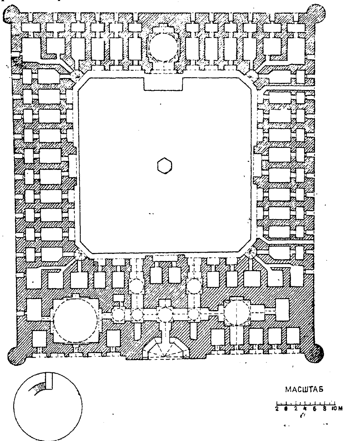
Рис. 23. План медресе Мухаммед-Амин-хана.
