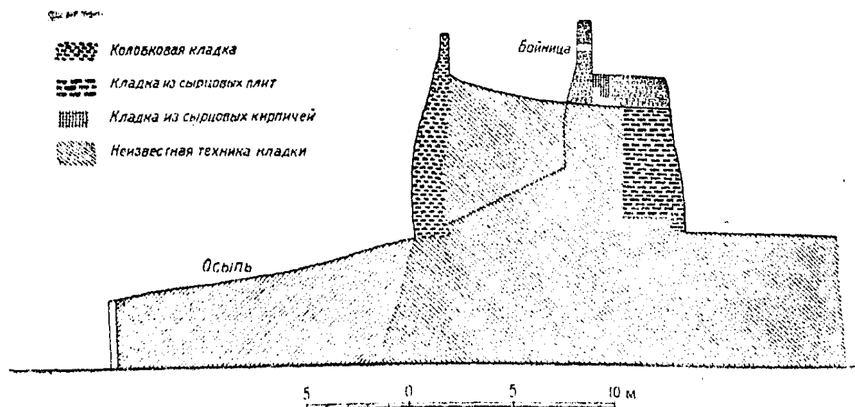
Рис. 4. Профиль башни и стены Ичан-Кала.
