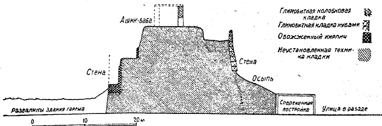
Рис. 7. Профиль Куны-Арка.
