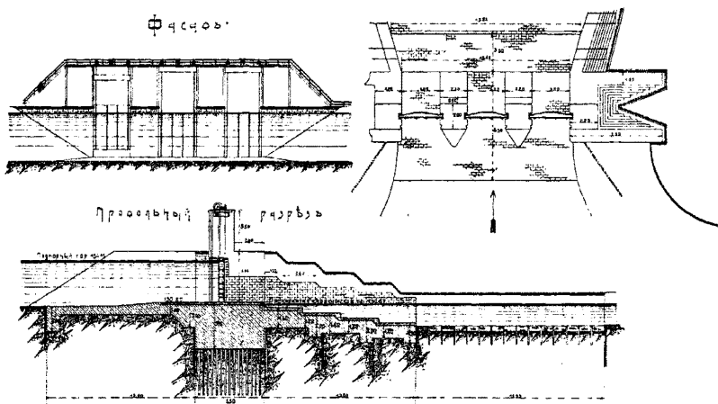
Черт. 32.
