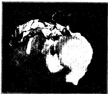
Фиг. 5. Сѣмянная коробка хлопка съ волономъ.
