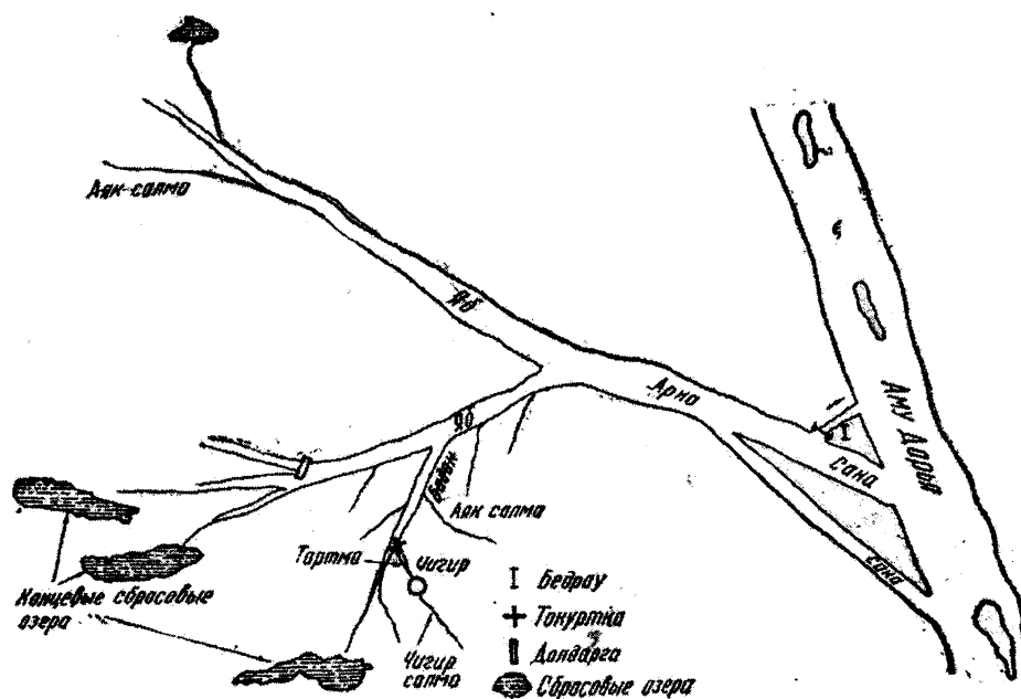
Рис. 3. Схема оросительной сети и сооружений в системе крупного канала в Хорезме. Гулямов Я.Г. История орошения Хорезма с древнейших времен до наших дней. Изд-во АН УзССР, Ташкент, 1957, 244с.
