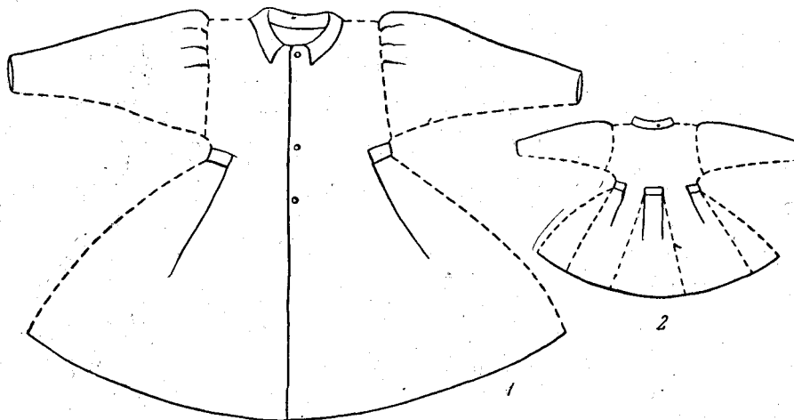
Рис. 5. Выкройка халата якутского покроя. 1 — вид спереди; 2 — вид сзади
