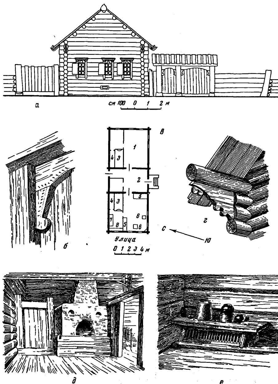
Рис. 6. Дом И. И. Ведерникова, д. Нижнее Суворово Братского района: а — фасад; б — деталь ворот; в — план: 1 — жилая изба, 2 — сени, 3 — печь, 4 — голбец, 5 — кровать, 6 — стол, 7 — залавок, 8 — лавка; г — повал; д — печь с голбцем; е — залавок
