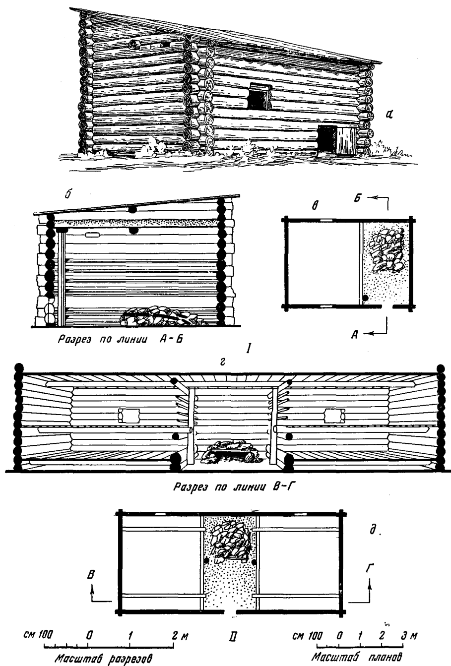
Рис. 9. Риги Братского района: I — односадная рига, д. Наратаи: а — общий вид, б — разрез, в — план; II — двухсадная рига, д. Романово: г — разрез, д — план
