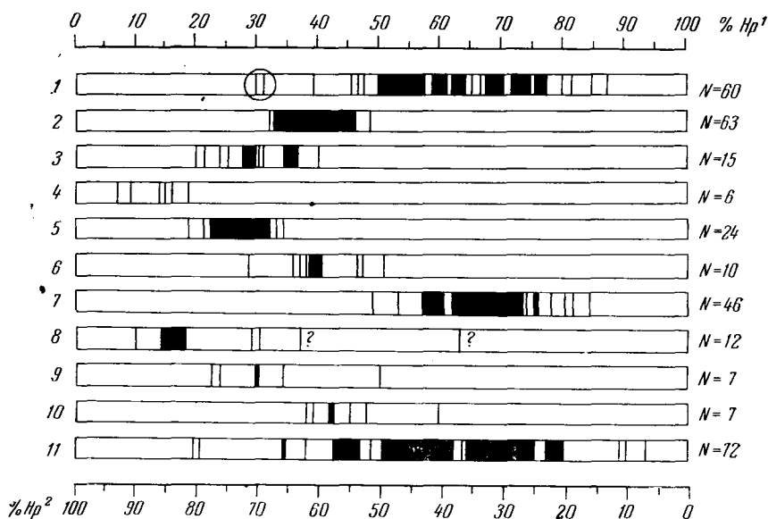
Рис. 4. Графики распределения частот гена Hr^1 . 1. Народы Африки (кругом обведены бушмены); 2. Европеоиды Европы. 3. Европеоиды Азии. 4. Южно-индийская группа. 5. Монголоиды Азии. 6. Индонезийцы и микронезийцы. 7. Полинезийцы и меланезийцы. 8. Австралийцы-аборигены. 9. Эскимосы Америки. 10. Американцы Северной Америки. 11. Американцы Центральной и Южной Америки.
