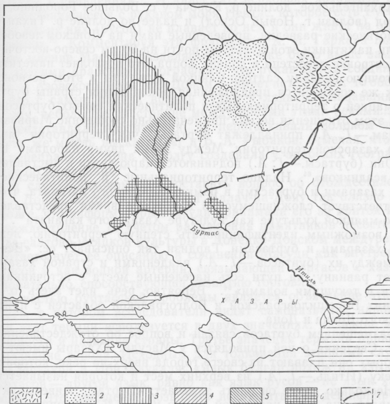
Археологические культуры лесостепной зоны Восточной Европы в VIII—X вв.: 1 — памятники волжских булгар; 2 — памятники мордвы и муромы; 3 — памятники вятичей на Оке; 4 — памятники северян (роменская культура); 5 — памятники донских славян (боршевская культура); 6 — памятники лесостепного (аланского) варианта салтово-маяцкой культуры; 7 — граница лесостепной зоны
