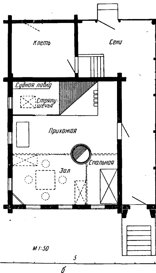
Рис. 10. Новый дом колхозника Блинова (постройка 1953 г.): а — внешний вид, б — план
