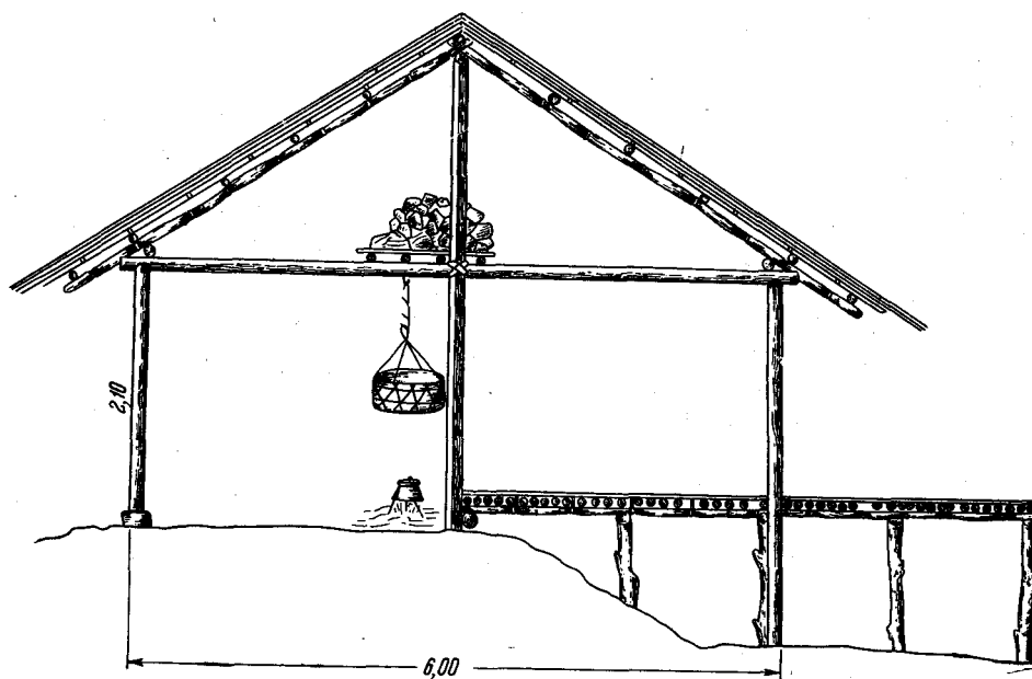
Рис. 6. Вертикальный разрез жилища ман
