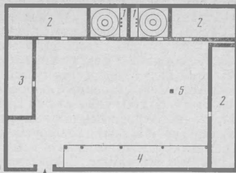
Рис. 4. Маслобойня (джувозхона) в Хуфаре: 1 — собственно джувозхона, 2 — стойло для быков ( гаухона ), 3 — стойло для лошадей ( аспхона ), 4 — навес с кормушками ( чуптора ), 5 — привязь для лошади ( яккамех )
