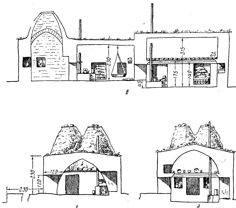
в — разрез по АБ; г — разрез по ВГ; д — разрез по ДЕ
