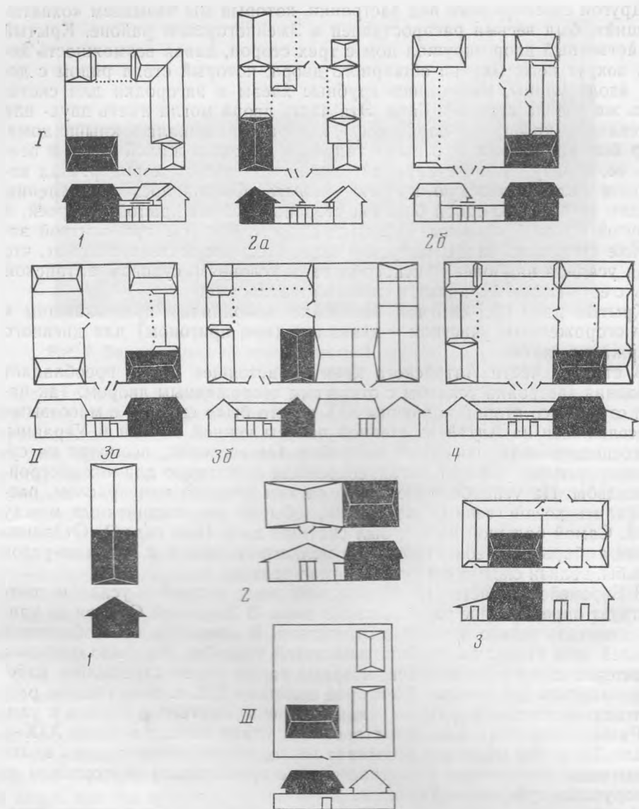
Рис. 3. Схематические планы застройки усадьбы I. Замкнутая застройка: I — нераздельная усадьба; 2 — двухчастная усадьба: а) с пригоном сзади ограды, б) с пригоном сзади дома; 3 — двухчастная усадьба: а) с пригоном сбоку от ограды, б) с пригоном сбоку от дома; 4 — двухчастная усадьба с задворьем. II. Слитная застройка: 1 — одно-рядная, 2 — двухрядная, 3 — охватывающая. III. Свободная застройка (На рисунке черной заливкой обозначен дом, контуром — хозяйственные постройки, контуром с пунктиром — навес.
