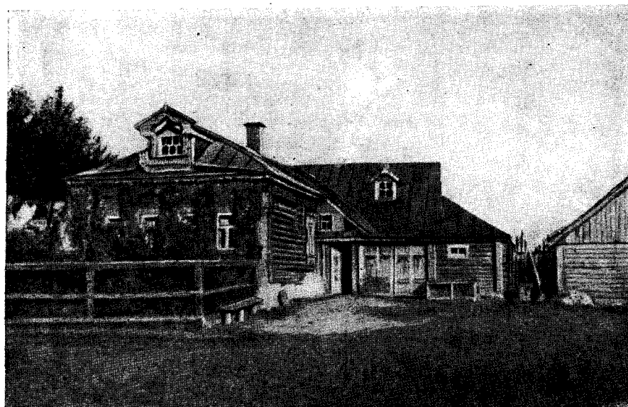
Рис 13. Поперечная застройка. Дом построен в 1925 г., двор — в 1948 г. Дер. Григорово Раменского района
