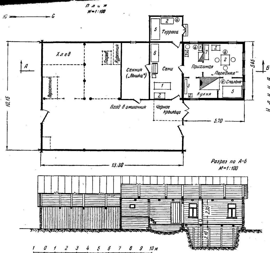
Рис. 15. План и разрез дома А. Н. Быковой, постройка 1947 г. Колхоз «Борец» Бронницкого района
