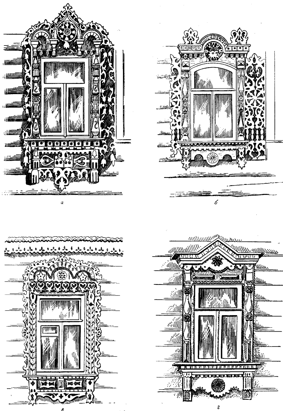
Рис. 5. Наличники окон в домах колхозников с. Гжель Раменского района: а, в — постройки 1924 г.; б — 1910 г.; з — 1923 г.
