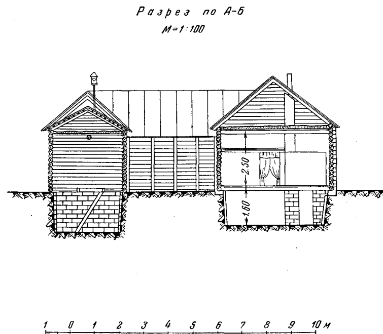
Рис. 10. План и разрез дома В. П. Архарова, постройки 1890 г. Колхоз «Борец», с. Рыболово, Бронницкого района
