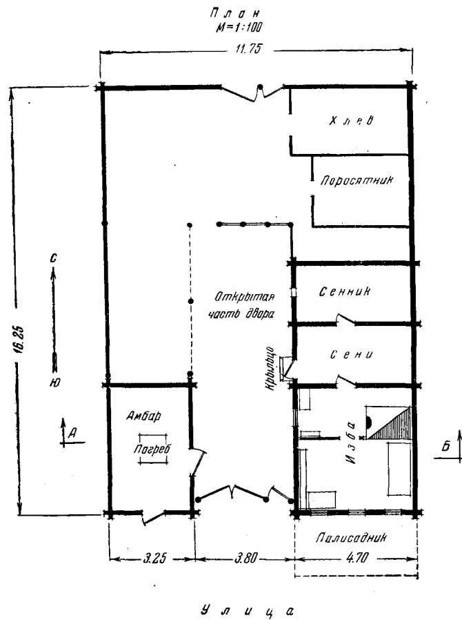
Рис. 10. План и разрез дома В. П. Архарова, постройки 1890 г. Колхоз «Борец», с. Рыболово, Бронницкого района
