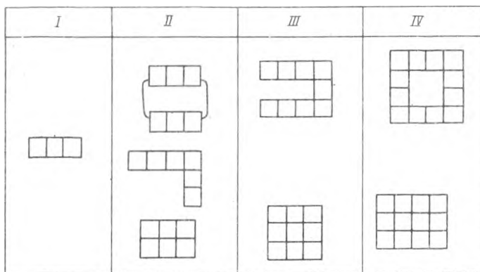
Рис. 1. Распределение традиционного корейского жилища (размеры даны в канов). I — 3; II — 6; III — 9; IV — 12 канов
