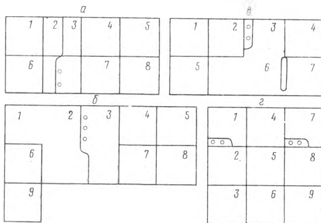
Рис. 3. Основные модификации двухрядных домов. а — восьмиканный дом с чонджуккан. 1 — хлев; 2 — кухня; 3 — чонджуккан; 4 — «верхняя» комната; 5 — дополнительная комната; 6 — помещение для крупорушки; 7 — кладовая; 8 — «нижняя» комната. б — десятиканный дом с чонджуккан. 1 — помещение для крупорушки; 2 — кухня; 3 — чонджуккан; 4 — «верхняя» комната; 5 — кладовая; 6 — «задняя кладовая»; 7 — дополнительная комната; 8 — «нижняя» комната; 9 — хлев. в — дом без чонджуккан. 1 — «нижняя» комната; 2 — «верхняя» комната; 3 — кухня; 4 — кладовая; 5 — гостиная комната; 6 — пондан, 7 — хлев. г — дом с тремя рядами комнат. 1 — кухня при гостевых комнатах; 2, 3 — гостевые комнаты; 4 — склад; 5 — кладовая; 6 — пондан; 7 — кухня при «большой» комнате; 8, 9 — «большая» комната
