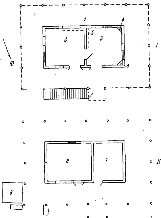
Рис. 3. Дом в поселке Чекишляр Гасан-кулийского района: I — верхний этаж; II — нижний этаж. I — саябан (навес); 2 — ашақы ой (западная комната); 3 — ёкарқы ой (восточная комната); 4 — полки; 5 — телер; 6 — жилая комната нижнего этажа; 7 — хозяйственное помещение; 8 — лар — цистерна для воды
