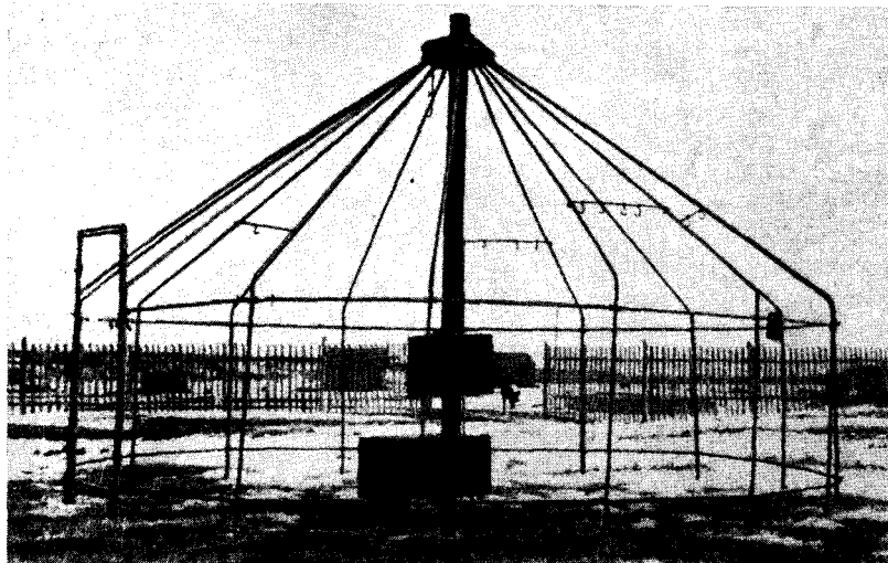
Рис. 6. Каркас сборно-разборного тордoха (чума) конструкции Л. Файко и И. Попова
