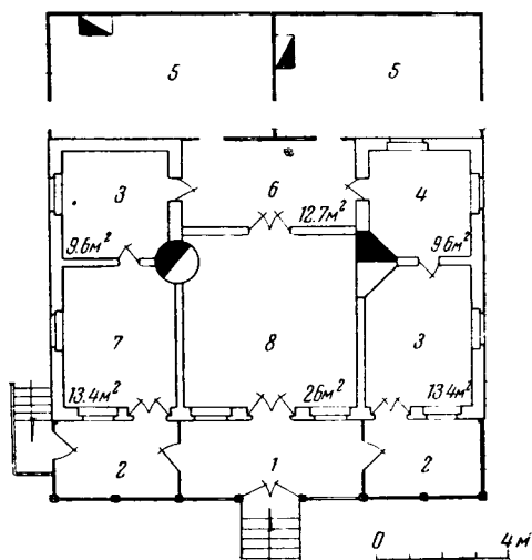
Рис. 6. Жилой дом К. Жвания, сел. Маяковский Маяковского р-на: 1, 2 — балконы; 3 — спальня; 4 — рабочая комната; 5 — пристройка; 6 — хозяйственный балкон; 7 — столовая; 8 — зал (по материалам Имеретинской этнографической экспедиции Ин-та истории АН ГрузССР, 1952 г.)
