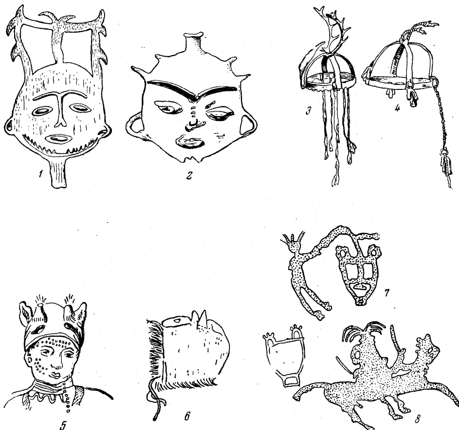
Рис. 10. Этнографические параллели к рис. 9 и датирующие археологические материалы: 1 — литое бронзовое изображение головы шамана, р. Илим (по Окладникову); 2 — литое бронзовое изображение головы шамана, р. Ангара (по Окладникову); 3 — корона бурятского шамана (по Агапитову и Хангалову); 4 — корона кетского шамана (по В. И. Анучину); 5 — тунгус в рогатой шапке, XVIII в. (по Георги); 6 — рогатая шапка якута (по Окладникову); 7, 8 — рисунки писаницы Кызыл-хая на р. Уйбате (по Апфельгрэн-Кивало)
