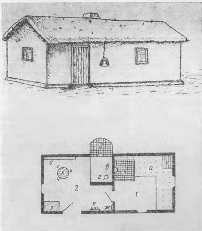
Рис. 2. Кухня (внешний вид и горизонтальный план): 1 — евь; 2 — кухня; а — пат-долма; б — фырын, соба; в — ба-жалык; г — очаг с железным треножником (сажак); д — летняя печь (фырын, кунтьор); е — бакрылык; ё — серген; ж — подвесной шкафчик (долма); з — уннух; и — юклюк; к — софра
