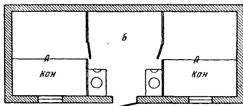
Рис. 2. Сравнительные планы ульчского и китайского жилища: 1 — ульчский дом хагду ; участки кана: а — пуску, б — допо, в — мали, г — панку, д — доу гело, е — бау гело, ж — гочи, з — аску, и — уйчу, помост для кормления собак; к — очаги; 2 — китайская фанза
