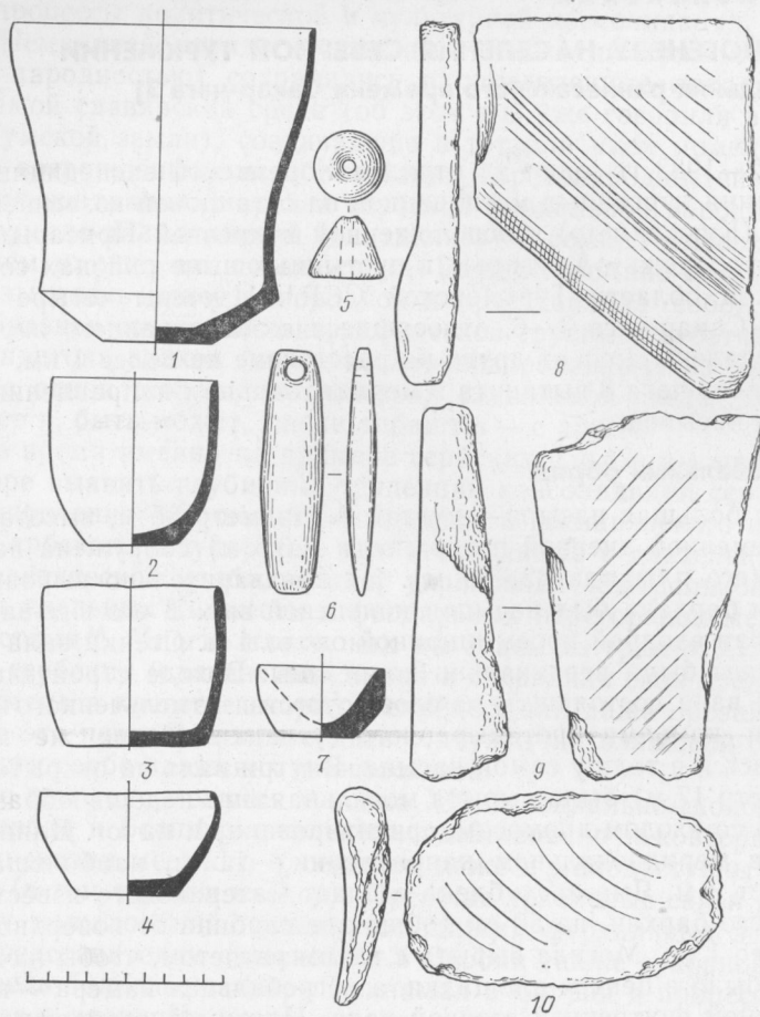
Рис. 1. Сопровождающий инвентарь из могильника Сакар-чага 3: 1 — гончарный кубок (курган 3); 2 — лепная чашка (курган 7); 3 — лепной сосуд (курган 7); 4 — лепная курильница (курган 4); 5 — глиняное пряслице (курган 2); 6 — каменный оселок (курган 3); 7 — каменная чашечка (курган 2); 8—10 — каменные зернотерки (курганы 1, 2)
