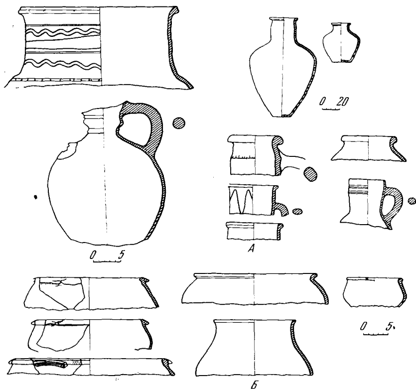
Рис. 2. Керамика с поселений нижнего Узбоия: А — гончарная посуда; Б — лепная посуда
