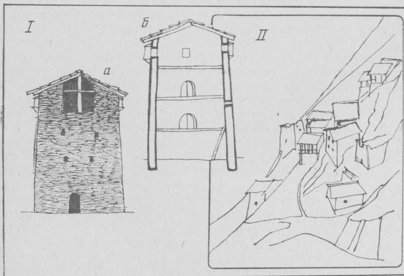
Рис. 3. Тушети. I. Дом-крепость из с. Чиги (рис. 1930-х годов): а — фасад, б — разрез. II. Общий вид части села Дочу (рис. 1984 г.)
