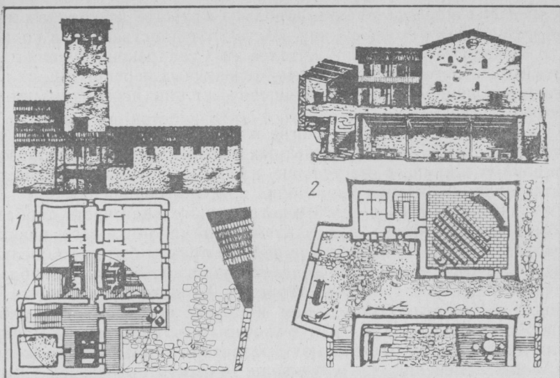
Рис. 4. Проекты приспособления сванских жилых комплексов под здания общественного назначения: 1 — проект гостиницы, 2 — проект общественного здания многоцелевого назначения с кинолекционным залом (авторы: архитекторы Г. Метревели, В. Коридзе, Т. Сирбиладзе)
