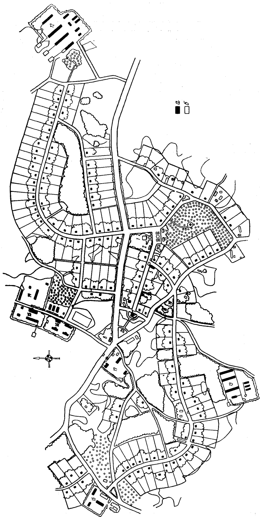
Рис. 5. План-проект поселка колхоза "Селия": а — запроектированные постройки; б — старые строения; 1 — клуб; 2 — столовая; 3 — магазин; 4 — многокомнатный жилой дом-общедитие; 5 — парикмахерская; 6 — детский сад; 7 — сельский совет; 8 — правление колхоза; 9 — баня-прачечная; 10 — амбулатория; 11 — почта; 12 — ферма крупного скота; 13 — ферма мелкого скота; 14 — птицеферма; 15 — конные дворы; 16 — склад; 17 — механические мастерские.
