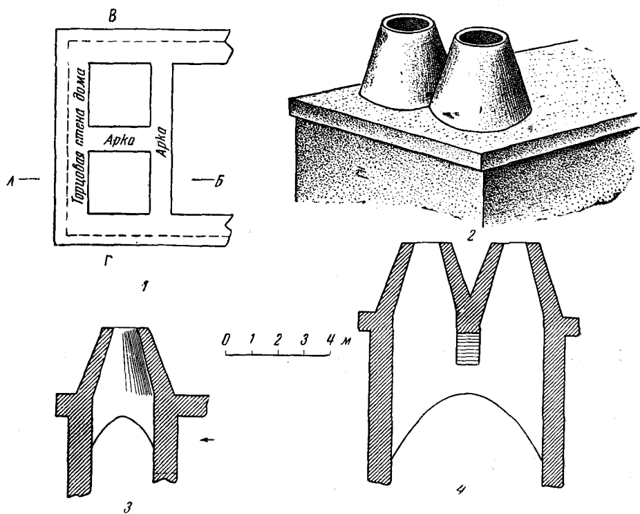
Рис. 6. Конструкция баджи аншеронского дома: 1 — план; 2 — общий вид; 3 — разрез по А — Б; 4 — разрез по В — Г
