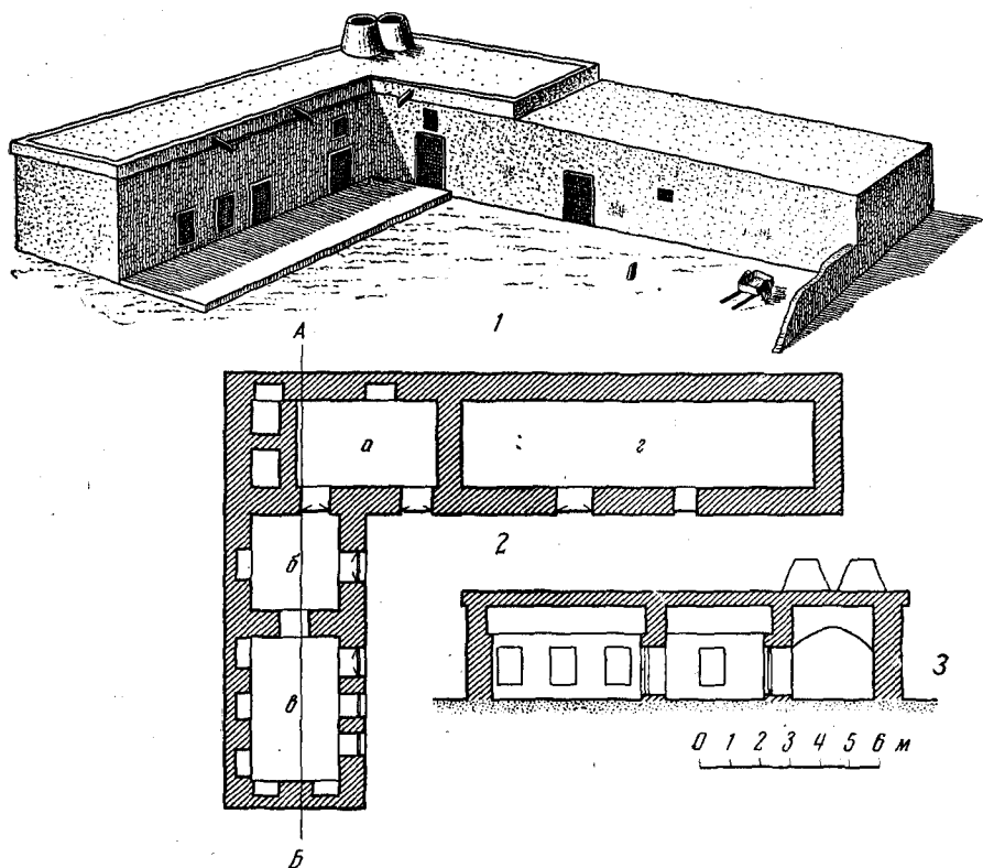
Рис. 5. Апшеронский дом (с. Балаханы Бакинского р-на Азербайджанской ССР): 1 — общий вид; 2 — план: а — общая комната, б — спальня, в — кузнецкая, г — хлев; 3 — разрез по А — Б
