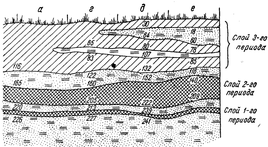
Рис. 3. Разрез культурных слоев Одоевского городища у основания вала (Буквы обозначают участки, цифры—глубину от поверхности в см)
