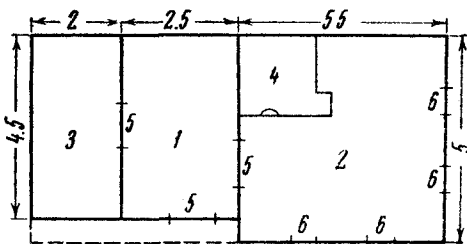
Фиг. 4. План хыжи гр. Г. (с. Керпни): 1 — сени, 2 — хыжа, 3 — «кліть», 4 — печь, 5 — двери, 6 — окна
