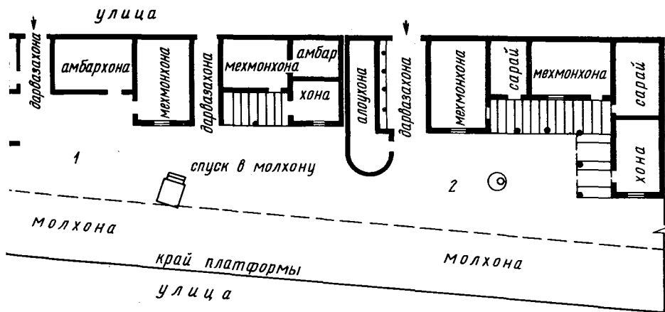
рис. 2. Планы жилых домов: 1 — Ходжи Саидназарова, 2 — Ниезахмеда Ибрагимова
