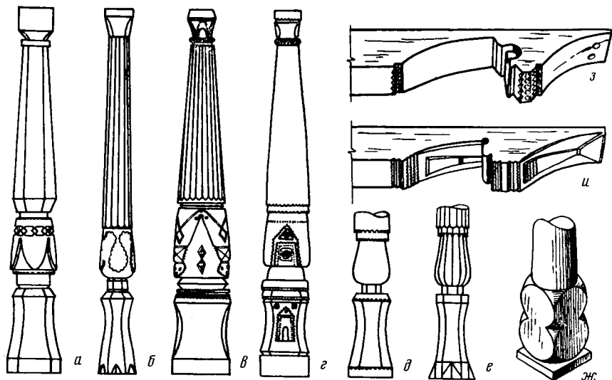
Рис. 5. Колонны Сурхандарьинской области: а — в мечети Суфи Алласта в Катта Вахшуваре, б — в мечети Дашнабада, в, г, д — в мечети Лючико в Хуфаре, е, жс — в мечети Мирзоб в Хуфаре; подбалки: з — в мечети Дашнабада, и — в мечети Лючико в Хуфаре
