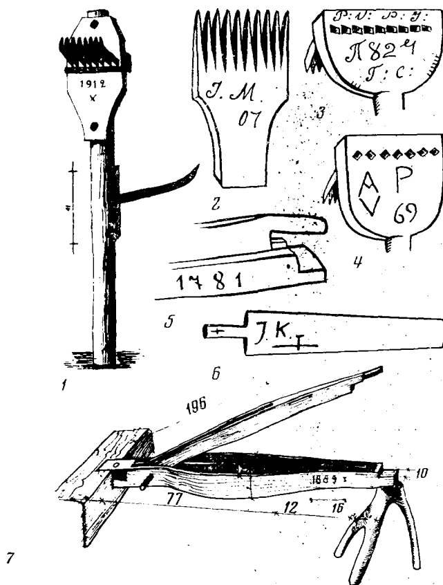
Рис. 1. Лīvõдžиекские орудия с надписями: 1 — столбовой драчок, 2 — бросальница, 3, 4 — драчок с рукояткой, 5 — фрагмент мялки, 6 — трепало, 7 — мялка
