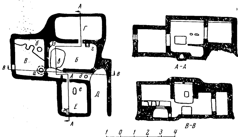
Рис. 1. План и разрезы восточного варианта старого традиционного жилища, дом Нунова Касима, к. Бидев (Ягноб); А — прихожая — куча ; Б — чистое отделение — канна ; В — очажное отделение — мур ; Г — кладовая — пстик ; Д — веранда — фарвор ; Е — помещение нового вида — хучра ; а — очаг — инкир , вкопанный в полу; б — возвышение с очагом на полу мур; в — ниша для дров в толще пола канны; г — яма для педалей ткацкого станка; д — яма-поглотитель — тахоратхона ; е — яма-зернохранилище — чагора ; ж — свето-дымовое отверстие — руча ; з — ниша-углубление в стене — чорах
