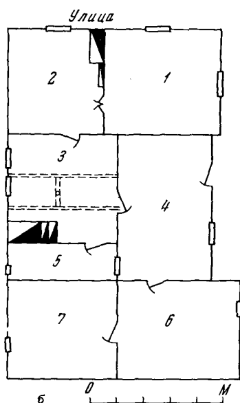
Рис. 5. Дом рабочего совхоза Я. Шнайнера в селе Октябрь- ское Карасукского района, по- строенный в 1954 г. а — внеш- ний вид; б — план; 1 — жилая комната, 2 — кухня, 3 — кухня- столовая, 4 — сени, 5 — кладо- вая, 6 — коровник, 7 — сеник (дровяник)
