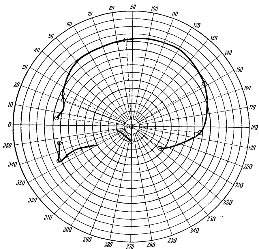
Рис. 3. «Круговой» график для вычисления среднего контура с интервалами 10° и 10 мм
