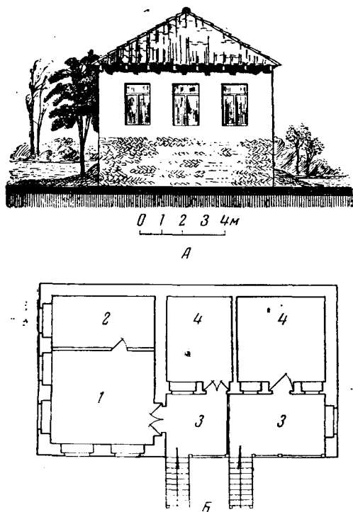
Рис. 9. Жилой дом В. Пичхнарашвили, с. Арбо Горийского р-на (по материалам Картлийской этнографической экспедиции, 1952 г.): А — фасад со стороны улицы; Б — план II этажа: 1 — гостиная; 2 — спальня; 3 — балкон; 4 — комната*
