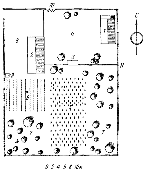
Рис. 8. Усадьба В. Джалабадзе, сел. Корди Горийского р-на: 1 — жилой дом; 2 — кухня; 3 — кукурузник и свинарник; 4 — двор; 5 — виноградник; 6 — огород; 7 — плодовый сад; 8 — пашня; 9 — уборная; 10 — главный вход (по материалам Картлийской этнографической экспедиции Ин-та истории ГрузССР 1952 г.)
