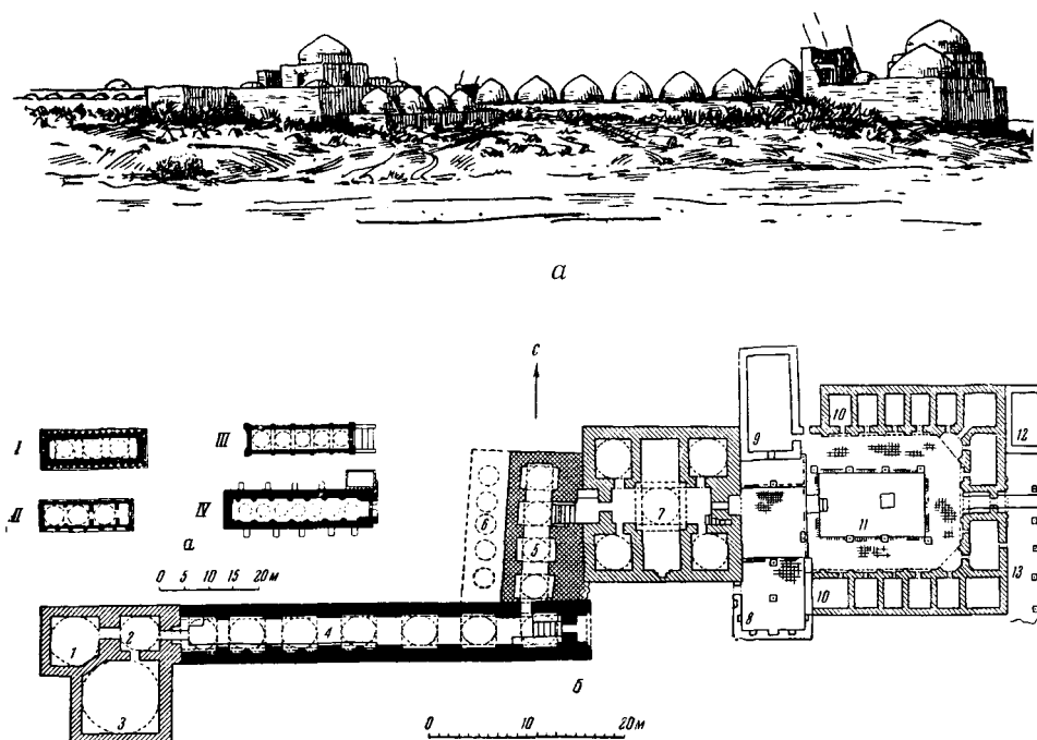
Рис. 1. Ансамбль Исмаут-ата: а — общий вид с северо-западной стороны; б — генеральный план (обмер автора): 1 — мазар «святого» Исмы; 2 — тилау-хана; 3 — корихана, 4 — даш-куча; 5 — коридор; 6 — захоронения хивинского духовенства; 7 — мечеть; 8 — летняя мечеть; 9 — ош-хана; 10 — ханака; 11 — внутренний двор ханаки с айванами; 12 — дом шейха; 13 — внешний айван
