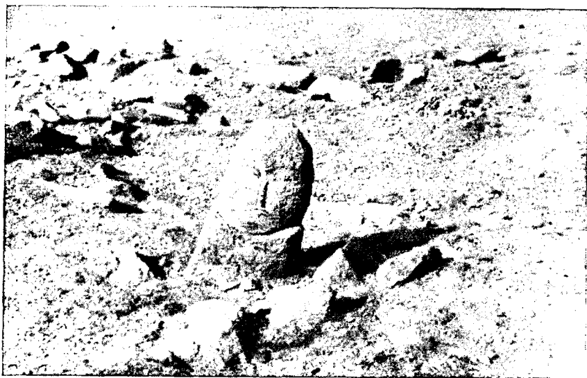
Рис. 3. Каменное изваяние у урочища Цайдам
