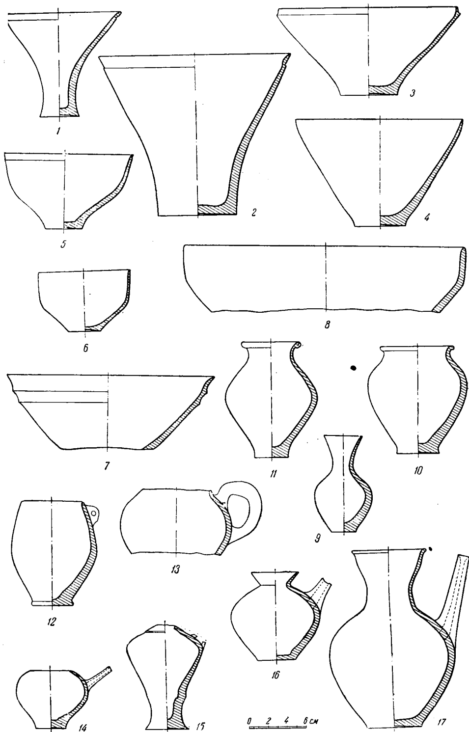
Рис. 5. Образцы керамики из зданий А и Б: 1—2—бокалообразные сосуды; 3—8—чаши; 9—12—вазообразные сосуды; 13—17—кувшинообразные сосуды
