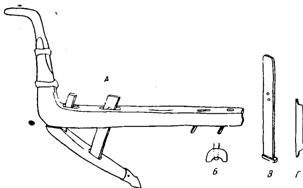
Рис. 9. Рало волове с приставной копыстью: А — рало; Б — сечение копысти; В — передняя снoз; Г — жабка; с. Староселье (№ 32184/267, 1/20 н/в)
