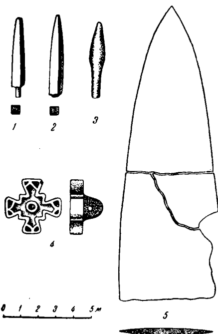
Рис. 12. Медные (бронзовые?) изделия: 1—3 — пробойники; 4 — печать; 5 — кинжал
