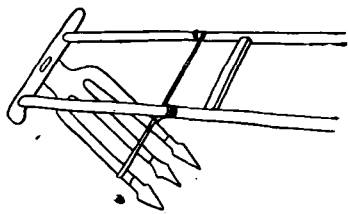
Рис. 30. Комстромская тройная соха (J. Falkowsky, Narzędzia rolnicze typu rylcowego, Lwow, 1934, рис. 73)
