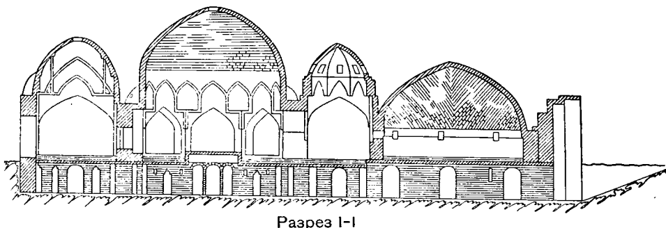
Разрез I-I
