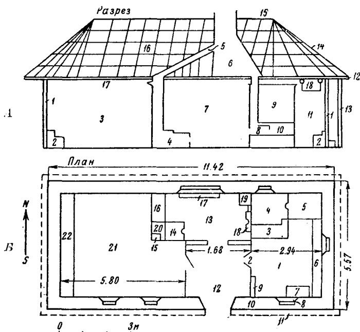
Рис. 3. Новый дом С. И. Кожухарь: А — разрез: 1 — перете; 2 — канапкэ; 3 — касэ чей маре; 4 — плитэ; 5 — ходжякул мик; 6 — ходжякул маре; 7 — кумната; 8 — ватра; 9 — собэ; 10 — кутерь; 11 — кэмара; 12 — стрешинэ; 13 — стылп; 14 — лецурь; 15 — каприорь; 16 — аконоремынт; 17 — под; 18 — кульмэ. Б — план: 1 — кэмара; 2 — уша; 3 — собэ; 4 — пе кутерь; 5 — пат; 6 — канапкэ; 7 — ладэ; 8 — ферястрэ; 9 — котинец; 10 — перетеле; 11 — приспа пе фарэ; 12 — тиндэ; 13 — кумната; 14 — духоукэ; 15 — трубэ; 16 — пат; 17 — масэ; 18 — кутерь; 19 — ватра; 20 — плитэ; 21 — касэ чей маре; 22 — канапкэ
