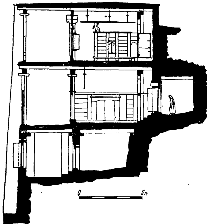
Рис. 4. Дом Гитино́. Поперечный разрез в современном состоянии. Верхняя жилая камера разрезана посередине, нижняя — по входу. В нижнем помещении показана поперечная ширма-перегородка более позднего происхождения
