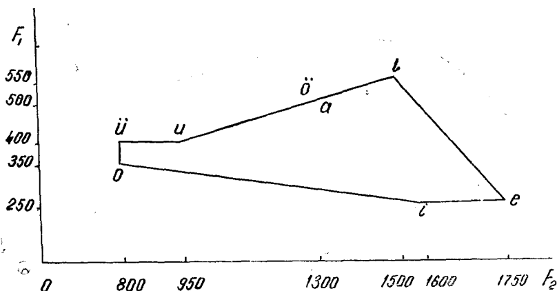
Рис. 2. Фигура расположения гласных турецкого языка, полученная в результате спектрального анализа.
