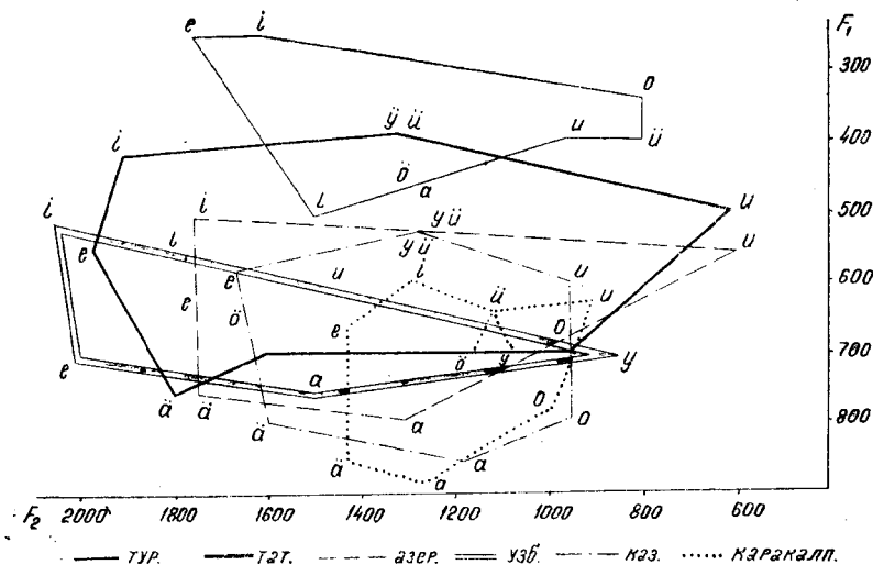
Рис. 4. Сравнительные рисунки расположения гласных турецких языков.
