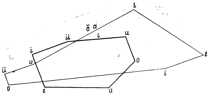
Рис. 3. Сравнительные рисунки расположения гласных в турецком языке традиционно и в результате спектрального анализа.
