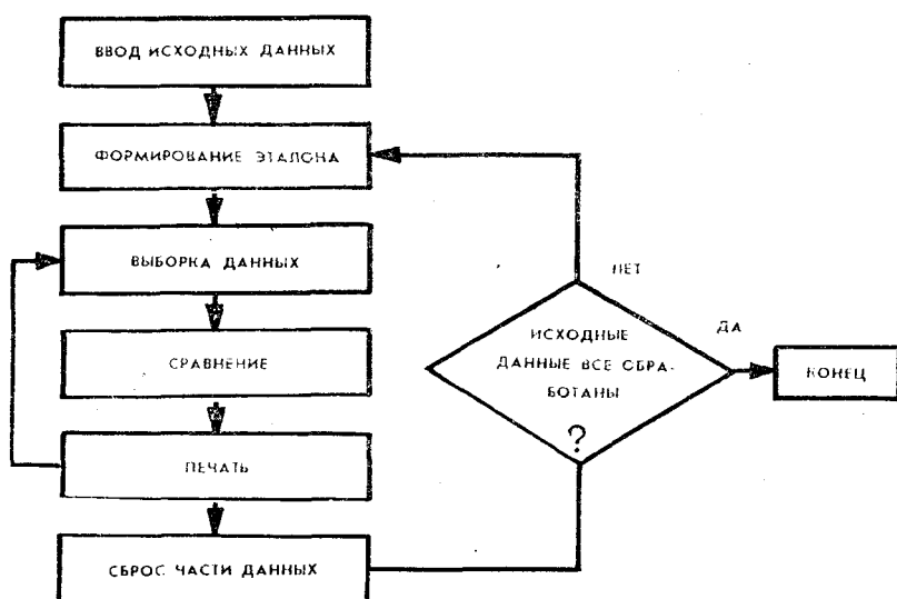
Функциональная схема алгоритма поиска родственных корней (основ).
