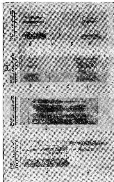
Рис. 4. Спектрограммы слов ăktă (I — д. И., II — д. А.), tără (д. А.), ăs (д. И.).
