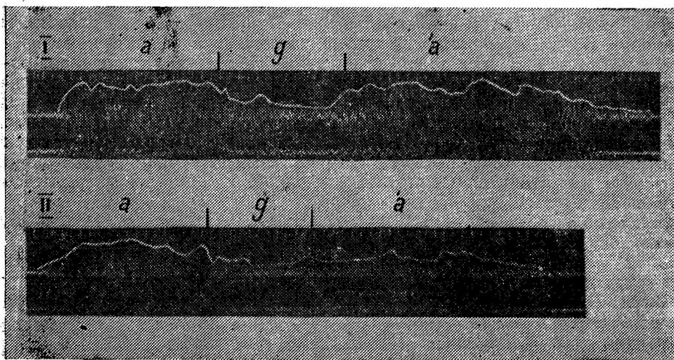
Рис. 2. Осциллограммы слова agá : I — д. Ч., II — д. Л.
