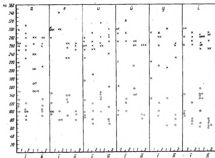
Рис. 1. Длительность безударных гласных в сравнении с длительностью ударных: o — указанный гласный находится в предударных слогах; x — ударные гласные в тех же словах; 1 — перед одиночными согласными; 2 — перед геминатами и сочетаниями согласных; I, II — дикторы.
