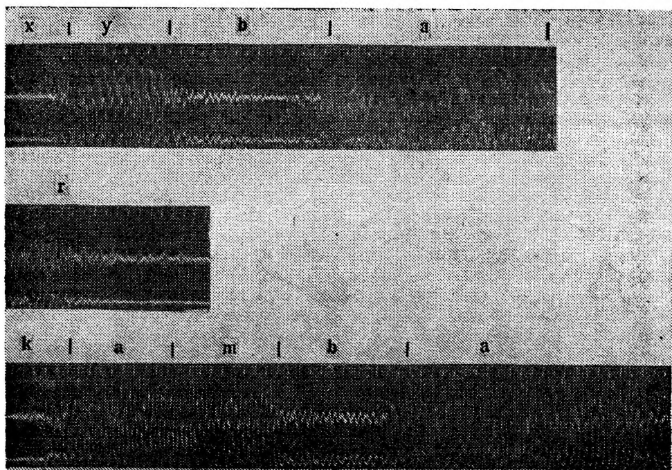
Рис. 5. Осциллограммы слов xuba'r , kamba' .
