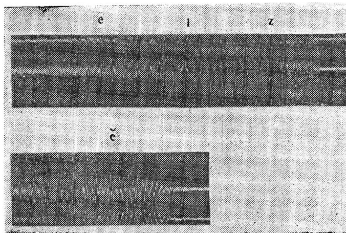
Рис. 1. Осциллограмма слова éze .
