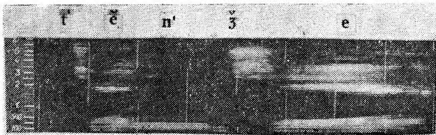
Рис. 4. Спектрограмма слова t'en'ze .
