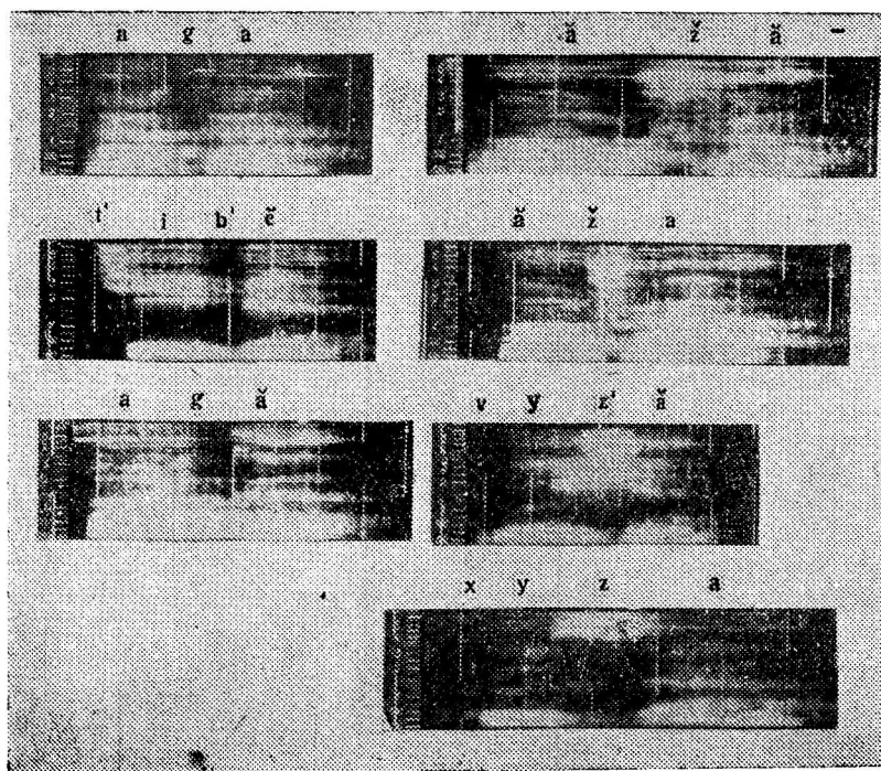
Рис. 3. Спектрограммы слов aga , t'ib'ë , agä , äžä , äža , vyž'ä , xuza .
