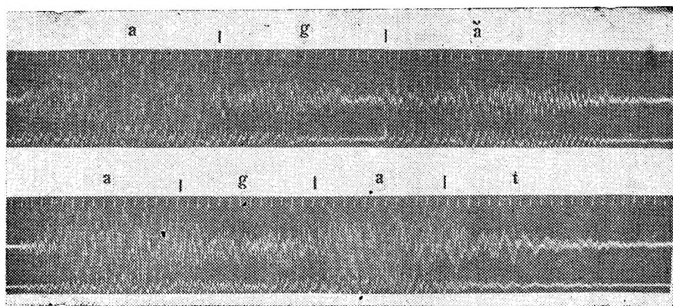
Рис. 2. Осциллограммы чувашского слова ágǎ и русского agái .
