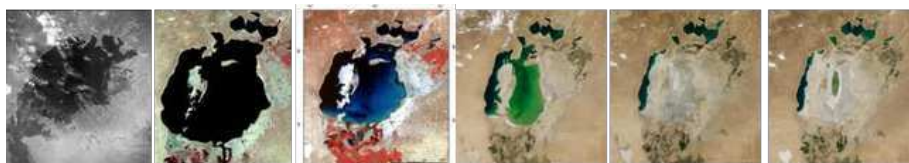
Рисунок 2.16. Снимки Аральского моря из космоса в период с 1964 по 2016 годы (источник: http://cawater-info.net )
