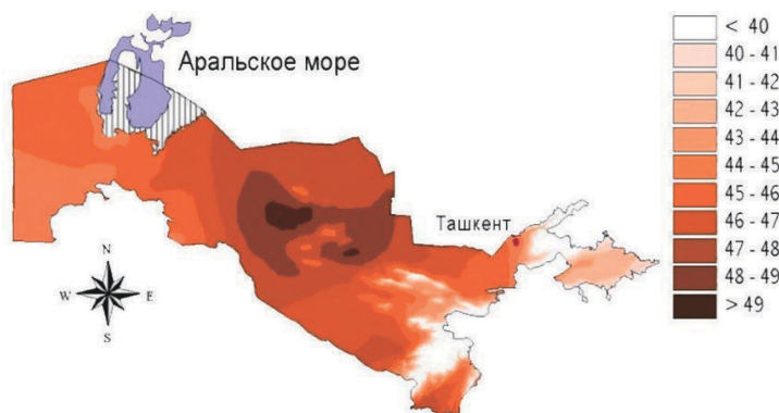
Рисунок 2.6. Температура в летний период (Третье национальное сообщение для Рамочной конвенции Организации Объединённых Наций об изменении климата Узбекистана, 2016)
